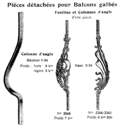
Feuille d'angle pour balcon galbé en fonte (idem). Col. AAM, Bruxelles.
