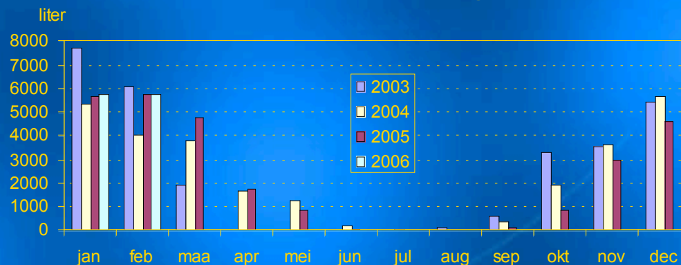
Verbruik verwarming
